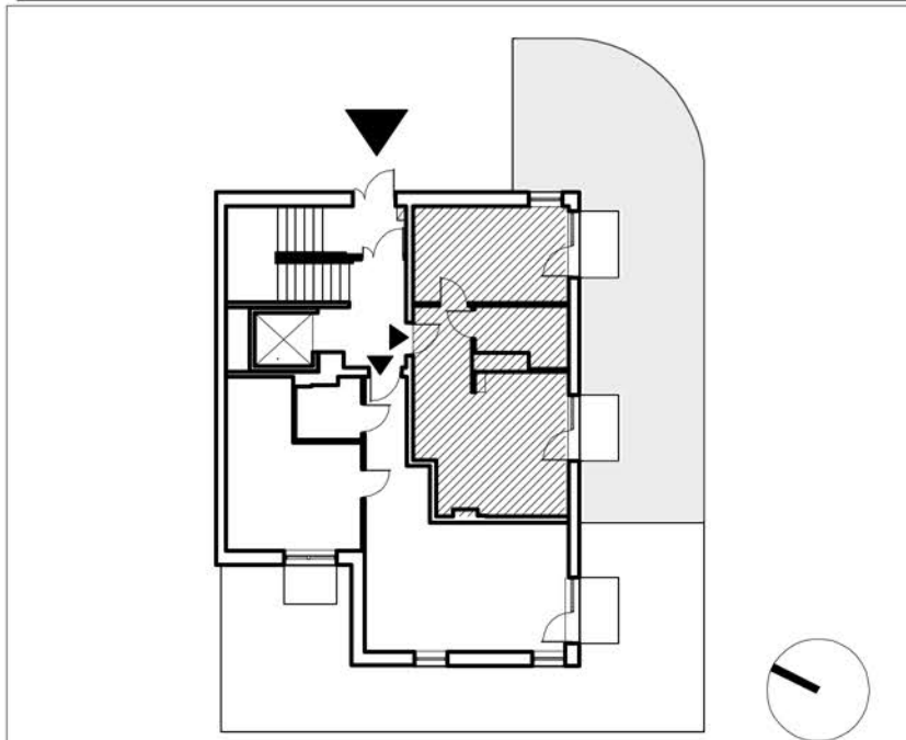
RZUT PARTERU BUD. 'B'
