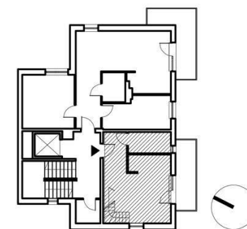
RZUT PIĘTRA I BUD. 'A'
