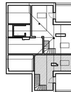
RZUT PODDASZA BUD. 'B'
