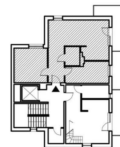
RZUT PIĘTRA I BUD. 'A'
