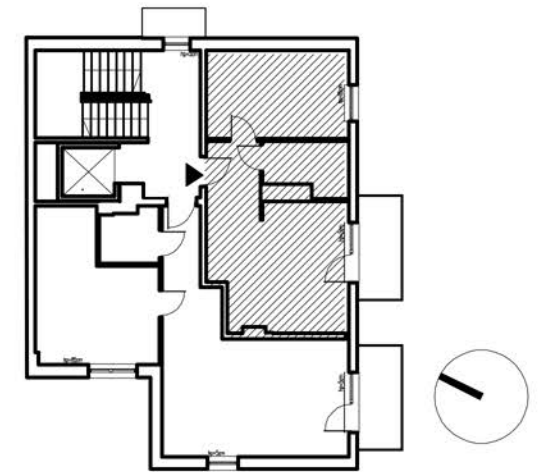
RZUT PIĘTRO I BUD. 'B'
