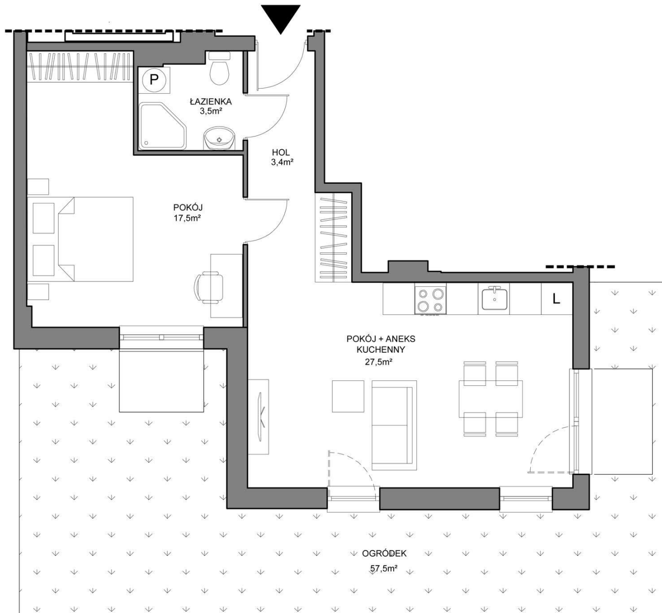
RZUT PARTERU BUD. 'B'
