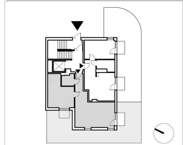
RZUT PARTERU BUD. 'B'
